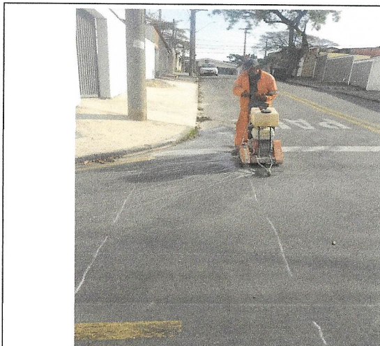
Demolição de pavimento na rua Matheus Haddad
