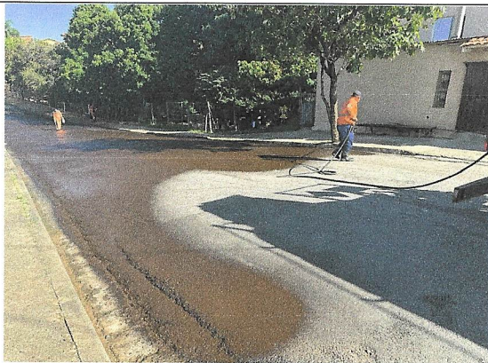
Imprimatura ligante na Rua Cesarpino Pires
